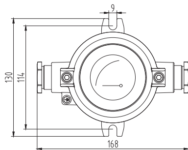
BZA5200-B Voltmeter/Ammeter
