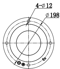
底盘尺寸
